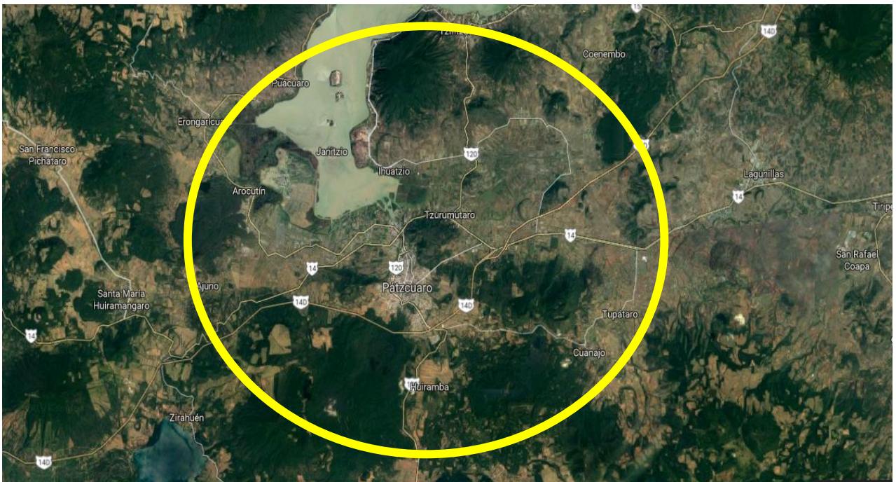
Zona de convergencia de Pátzcuaro.
